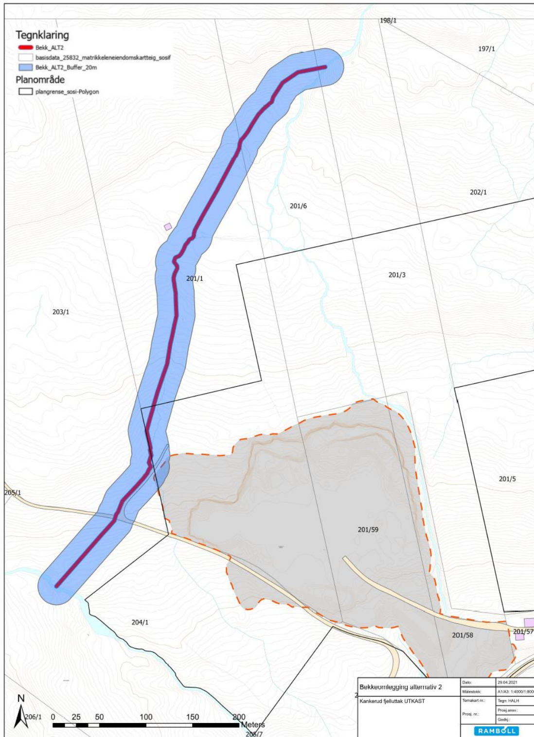
Utkast til plassering av bekk etter omlegging.
