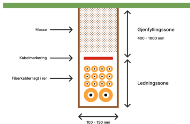
Kabelgrøft - Pløying
